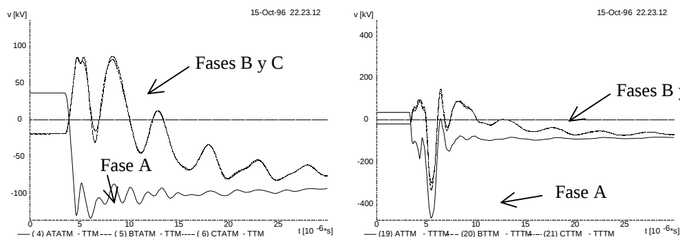
Figura 5: Tensiones en el transformador AT2 entre las fases A, B y C y el núcleo “at2” (izquierda) y tensiones en el transformador de tensión TT2 entre las fases A, B y C y el núcleo “tt2” (derecha), frente a un rayo de 10 kA, 1/20 \mu s y con sendos pararrayos en bornes de los transformadores.
